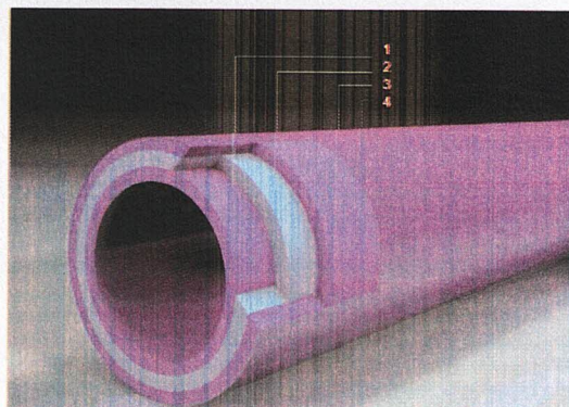
Vedere generală țeavă din PP-R aquatherm blue multistrat cu baieră de difuzie a oxigenului
