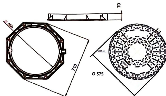
Vedere generală capac rotund pas 550mm
