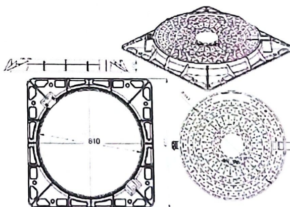
Vedere generală capac rotund pas liber 600mm
