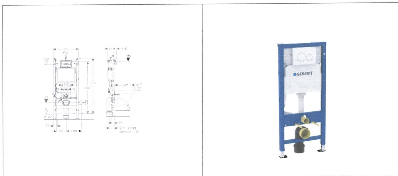
Modul Duofix pentru WC suspendat, cu rezervor incastat si clapeta de actionare
