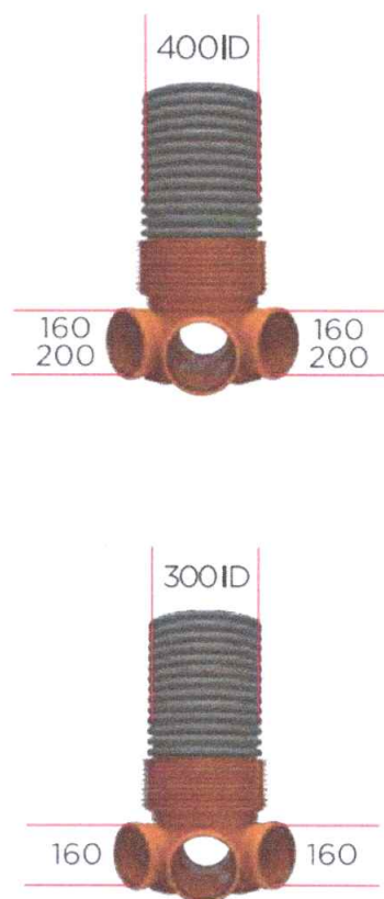
Fig 3 Cămine din element de bază din PP și coloană din teavă corugată PP
