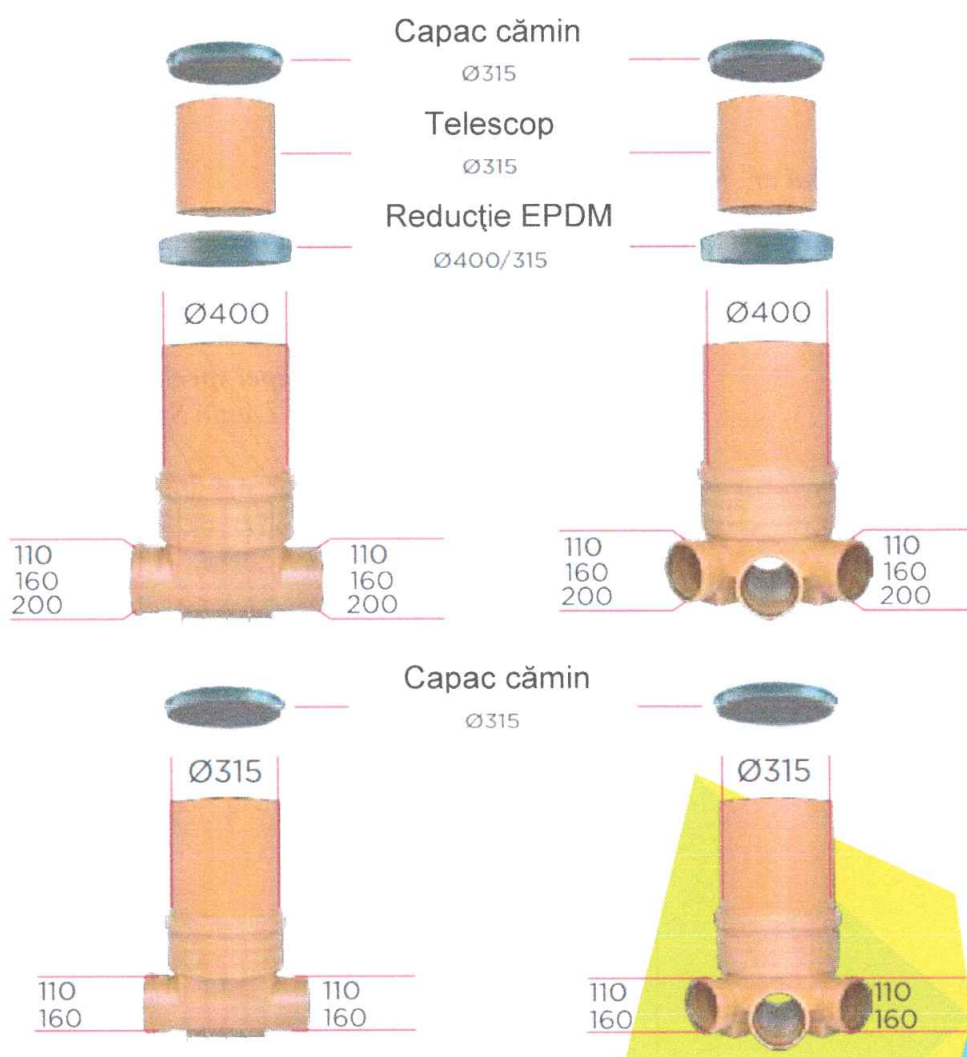
Fig. 2 Cămine din element de bază din PP și coloană din teavă lisă PP/PVC
