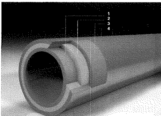
Vedere generală țeavă din PP-RCT aquatherm blue multistrat cu baie de difuzie a oxigenului
