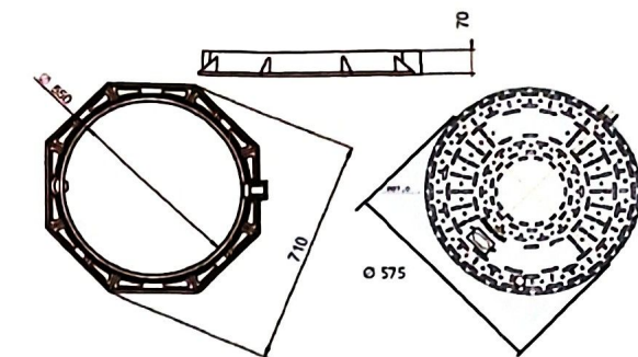
Vedere generală capac rotund pas 550mm
