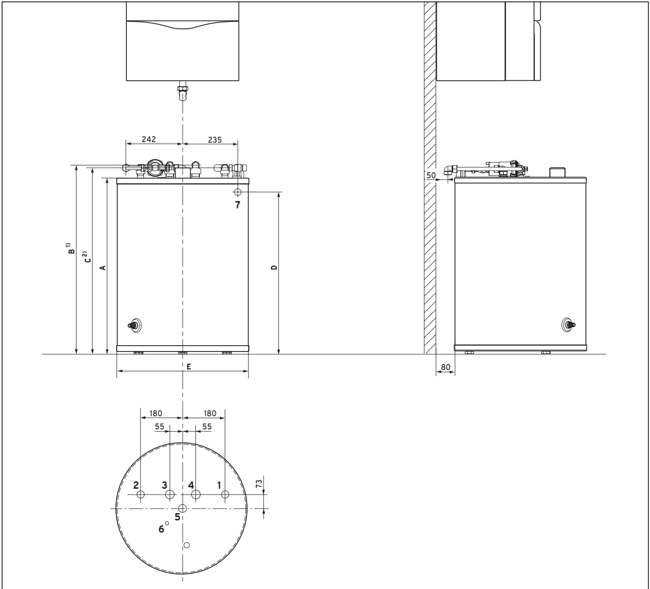
Şek. 4.2 Ebatları
