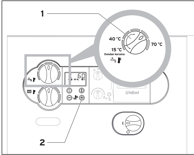
Şek. 3.1 Boyler sıcak su sıcaklığının ayarlanması
