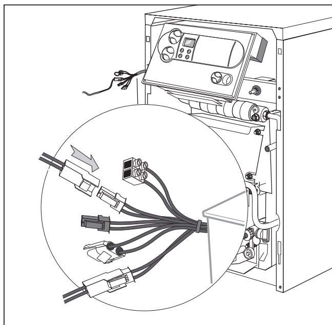
Fig. 4.4 Elektrisk installation
