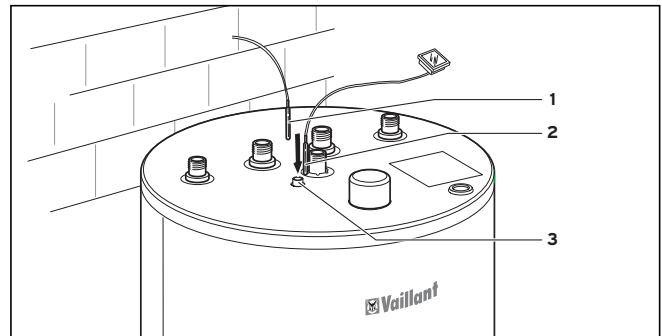
Fig. 4.3 Montarea senzorului
