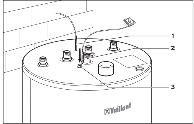
Şek. 4.3 Duyarganın montajı
