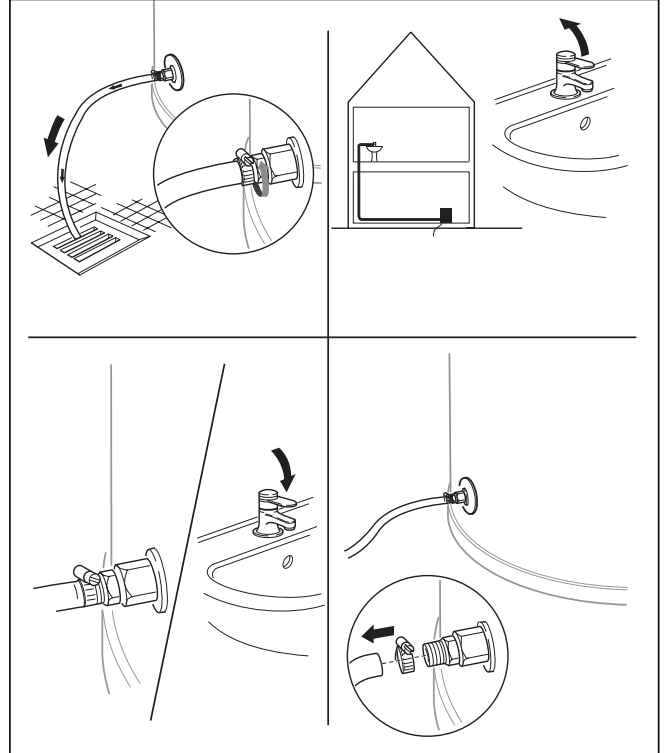
Şek. 6.1 Sıcak kullanma suyu boylarının boşaltılması
