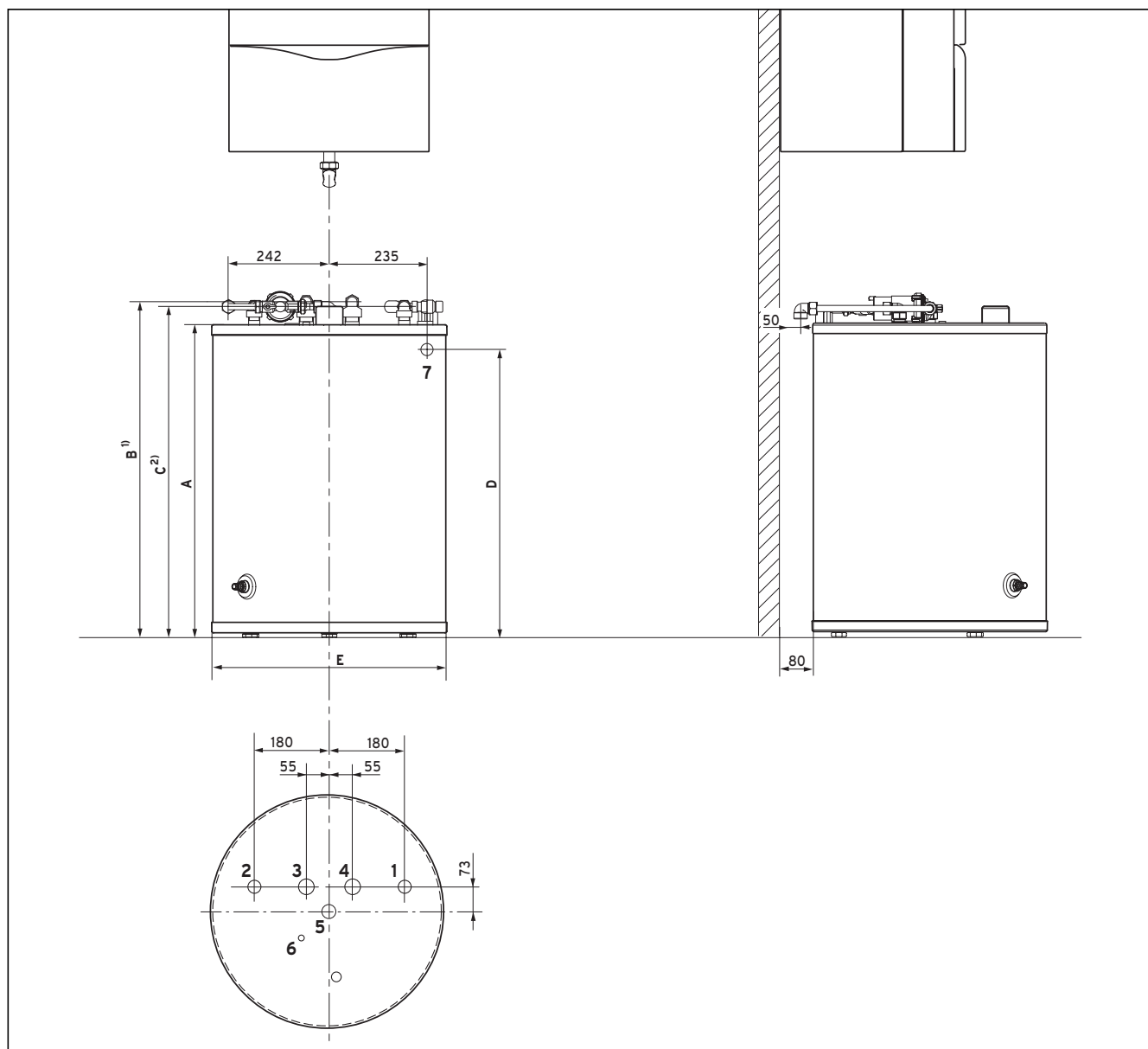
Fig. 4.2 Tilslutningsmål
