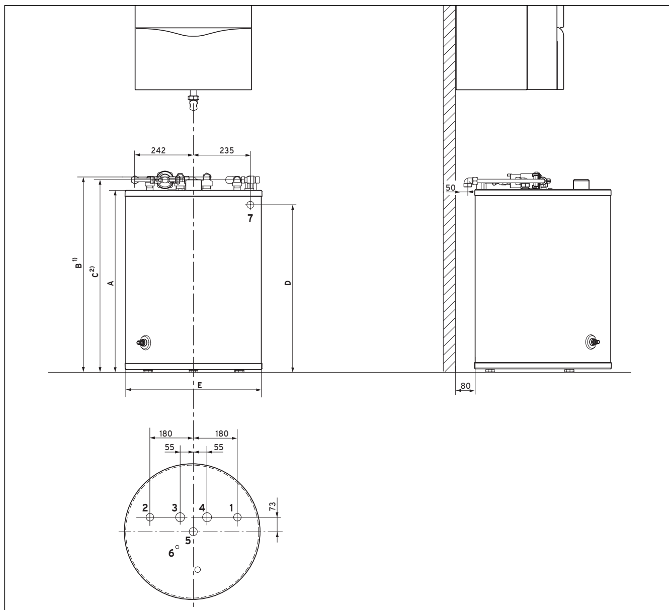
4.2 ábra: Méretraajz
