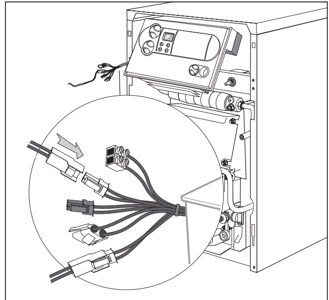
Şek. 4.4 Elektrik kablo bağlantıları
