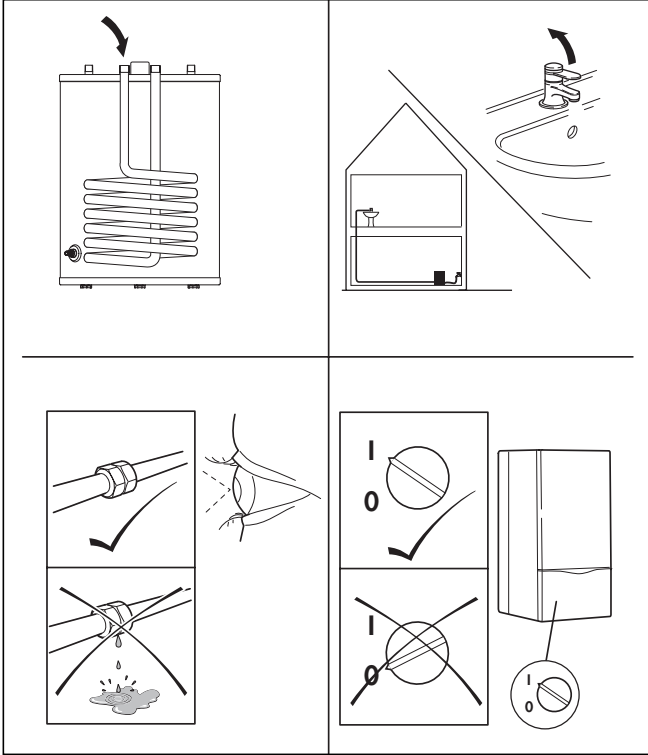
Şek. 5.1 Sistemin ilk devreye alınması
