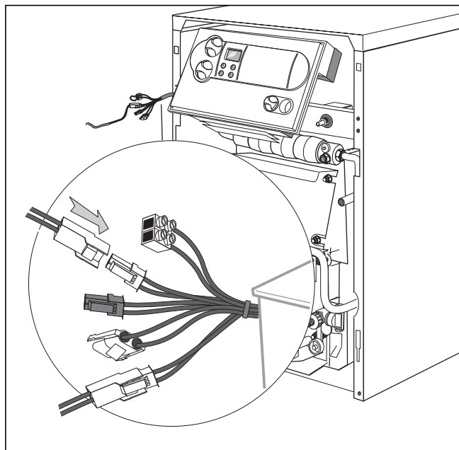
Obr. 4.4 Elektroinstalace
