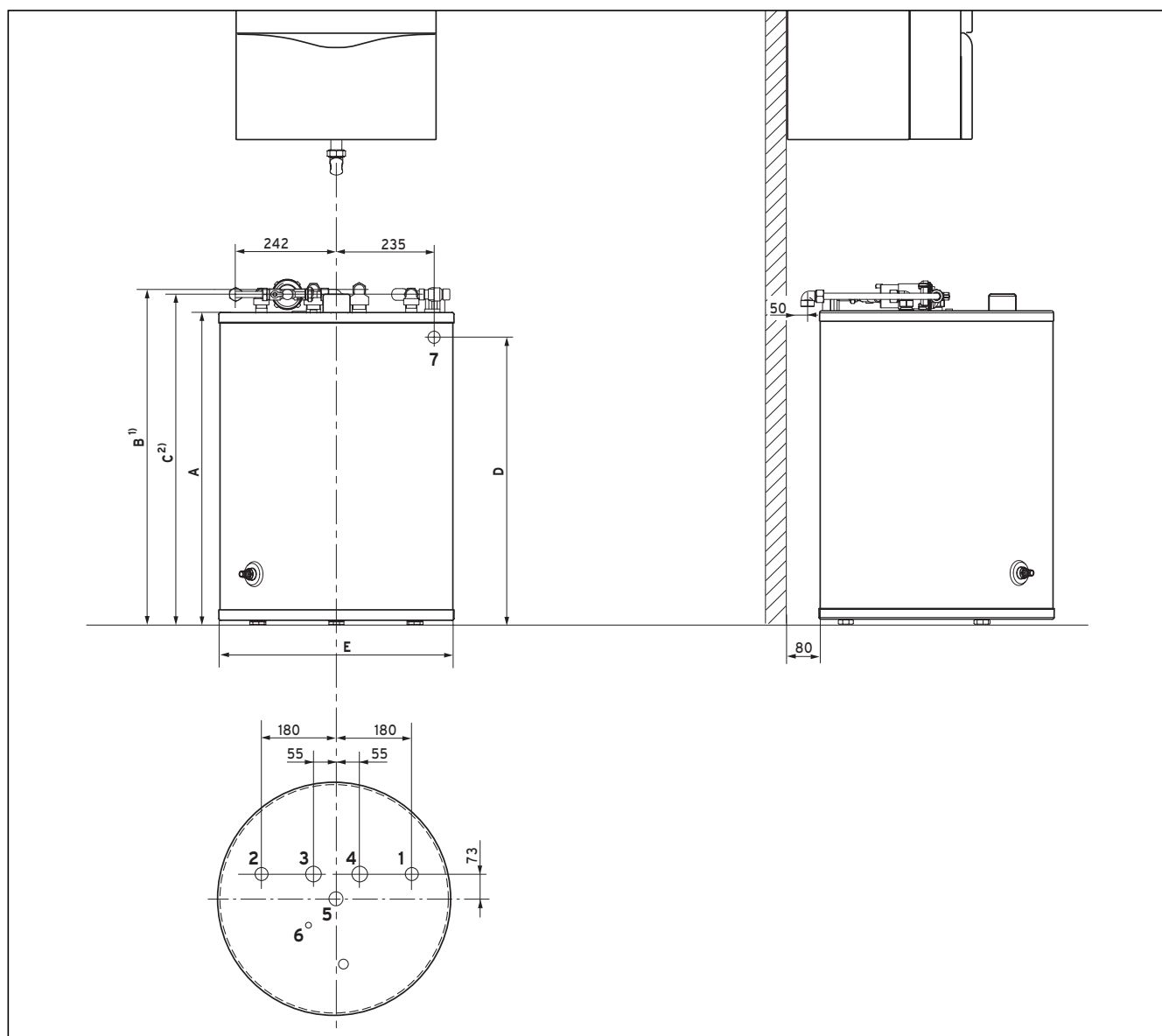
Fig. 4.2 Desen cotat
