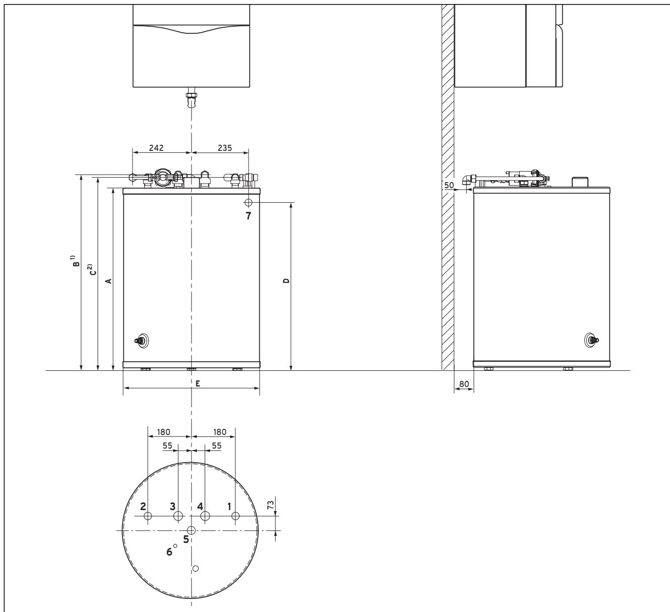
Fig. 4.2 Dimensions
