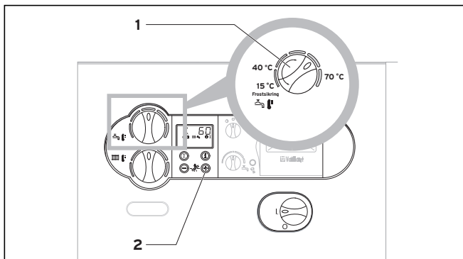
Afb. 3.1 Reservoirwatertemperatuur instellen
