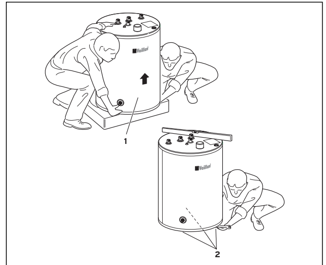
Şek. 4.1 VIH boylerinizi taşıması
