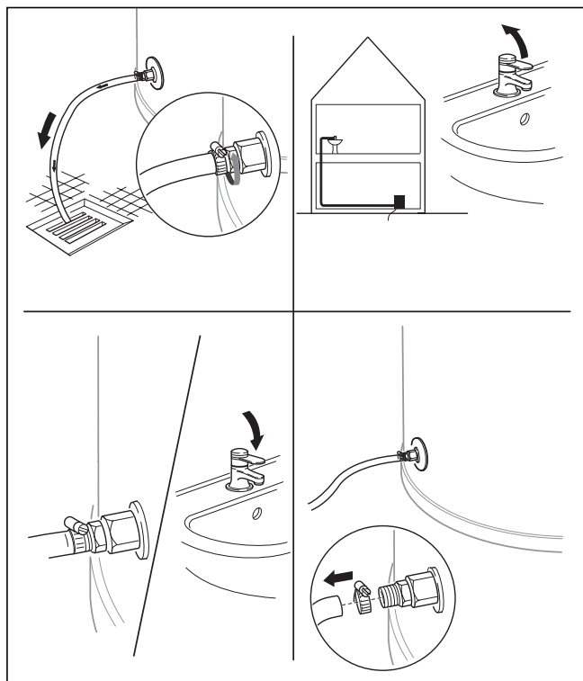
Fig. 6.1 Vaciado del acumulador de agua caliente
