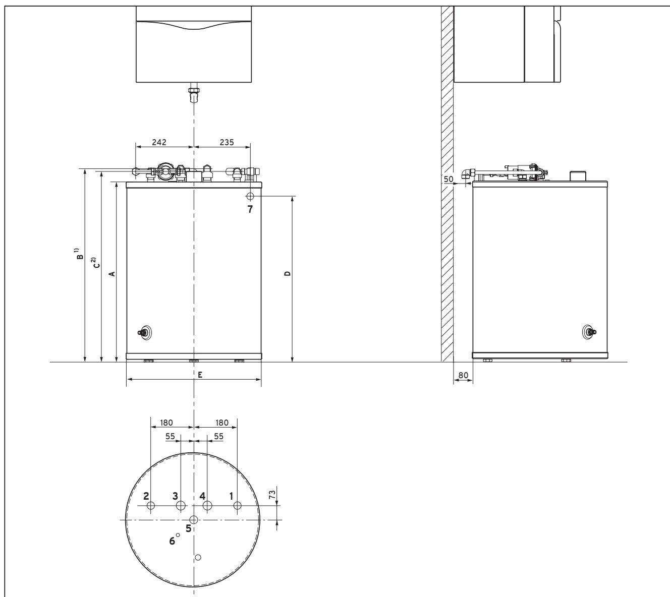
Rys. 4.2 Wymiary
