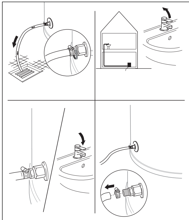
Fig. 6.1 Golirea boilerului de apă caldă menajeră
