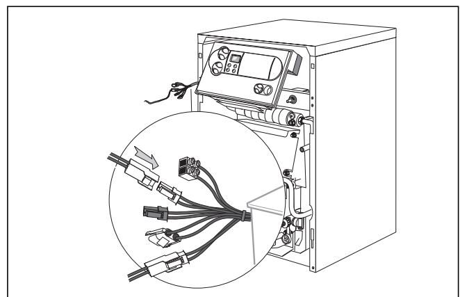
Fig. 4.4 Instalarea părții electrice
