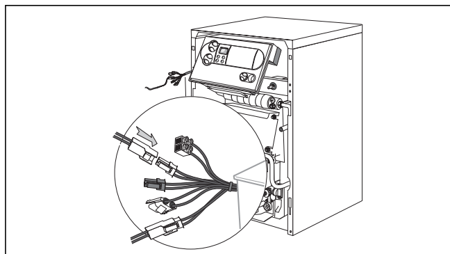
Fig. 4.4 Installation électrique
