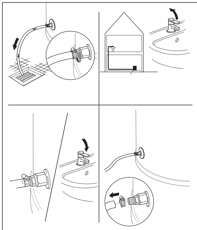
Obr. 6.1 Vyprázdnenie zásobníka teplej vody
