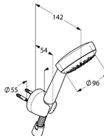
Desen dimensional
