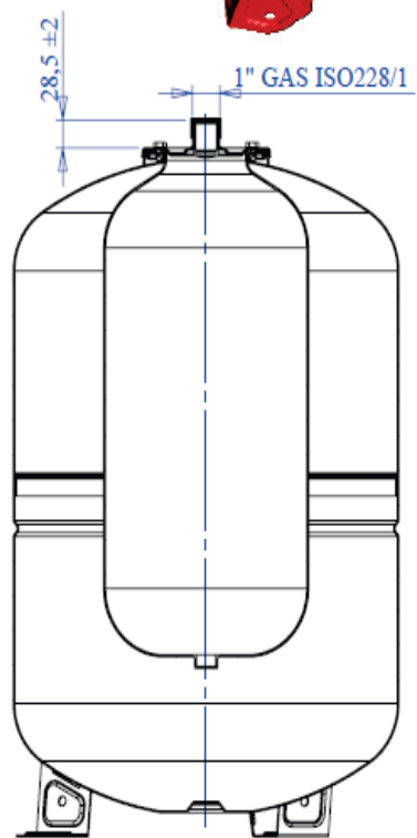
SECTIUNE C-C
