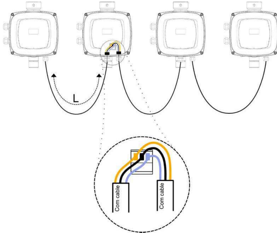
Figura 6: Exemplu de conexiune a comunicării multi inverter cu 4 dispozitive
