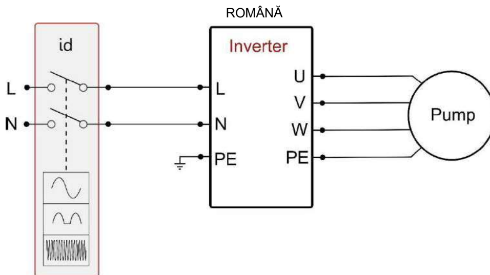
Figura 2a: Exemplu de instalare cu alimentare monofazică
