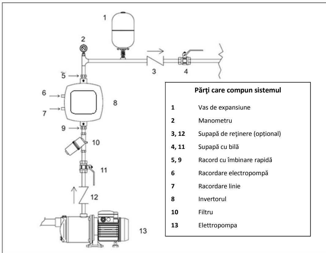
Figura 1: Instalație hidraulică
