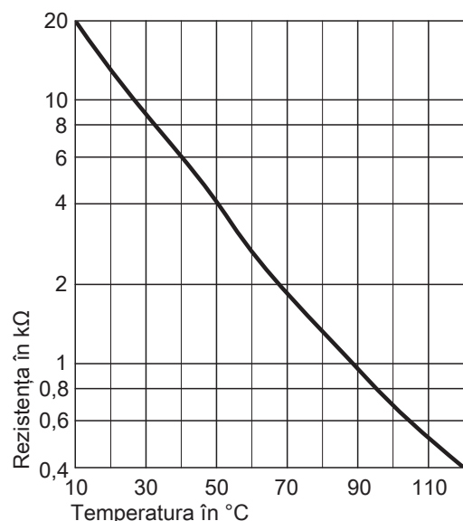
Fig. 50 Tipul senzorului: NTC 10 kΩ
