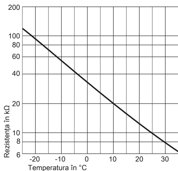
Fig. 46 Tipul senzorului: NTC 10 kΩ
