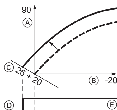
Fig. 36 Exemplul 1: Modificarea temperaturii nominale normale de ambianță de la 20 la 26 °C
