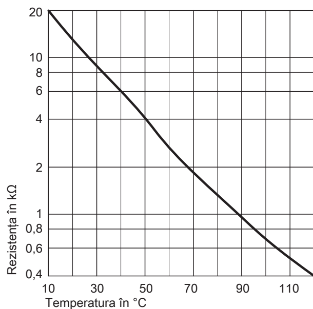
Fig. 53 Tipul senzorului: NTC 10 kΩ
