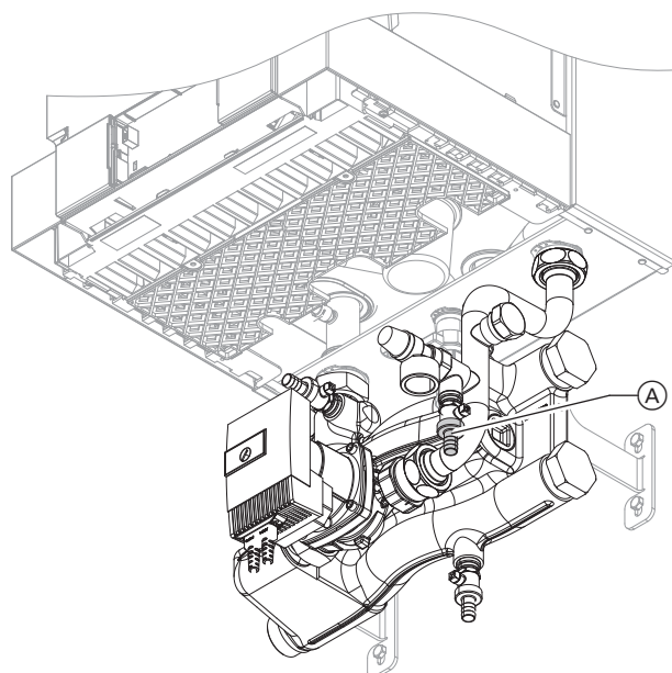
Fig. 20 Set de racordare cu preselector hidraulic integrat
