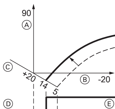
Fig. 37 Exemplul 2: Modificarea temperaturii nominale reduse de ambianță de la 5 °C la 14 °C
