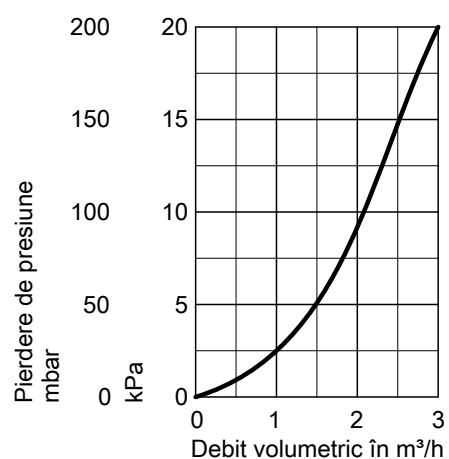
Diagrama pierderilor de presiune
