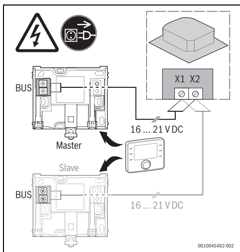
Fig. 6 Conectarea unităților de comandă la o unitate internă.
