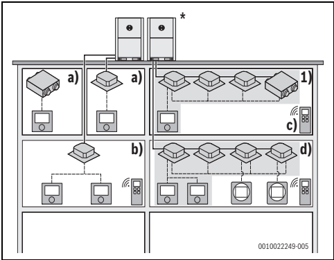
Fig. 1 Situații de utilizare ARC C-2/ARC H-2 (prezentare generală schematică; în figură nu este reprezentată cablarea/instalația de conducte efectivă)
