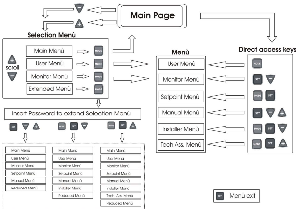
Figura 15: Schema posibilelor accesuri la meniuri
