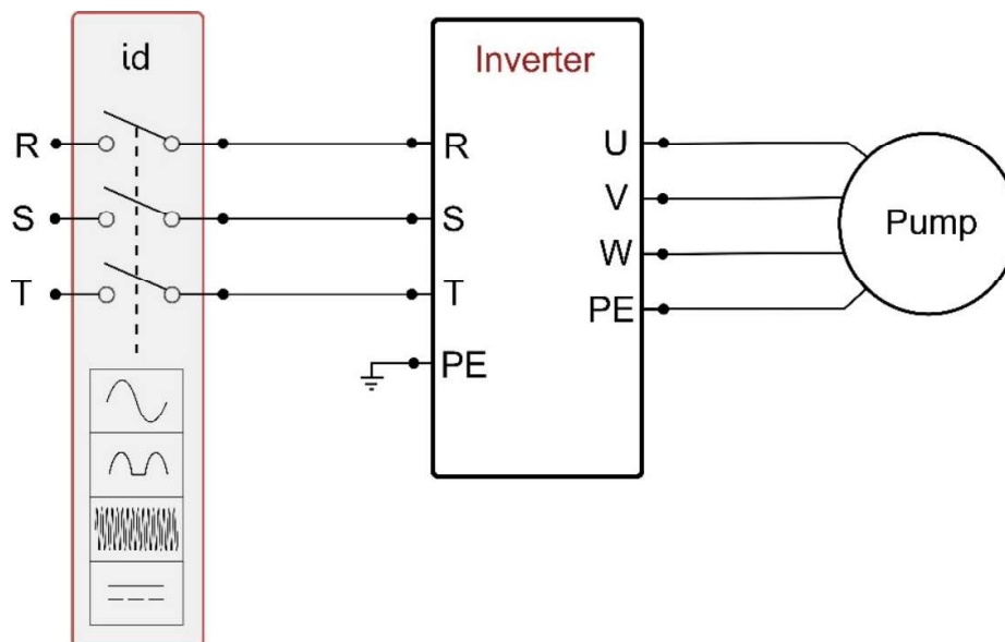
Figura 4b: Exemplu de instalare cu alimentare trifazică
