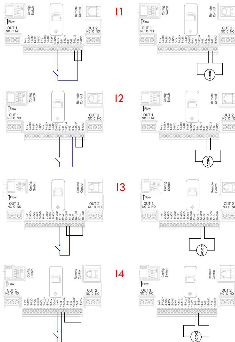
Figura 12: Exemplu de conectare a intrărilor
