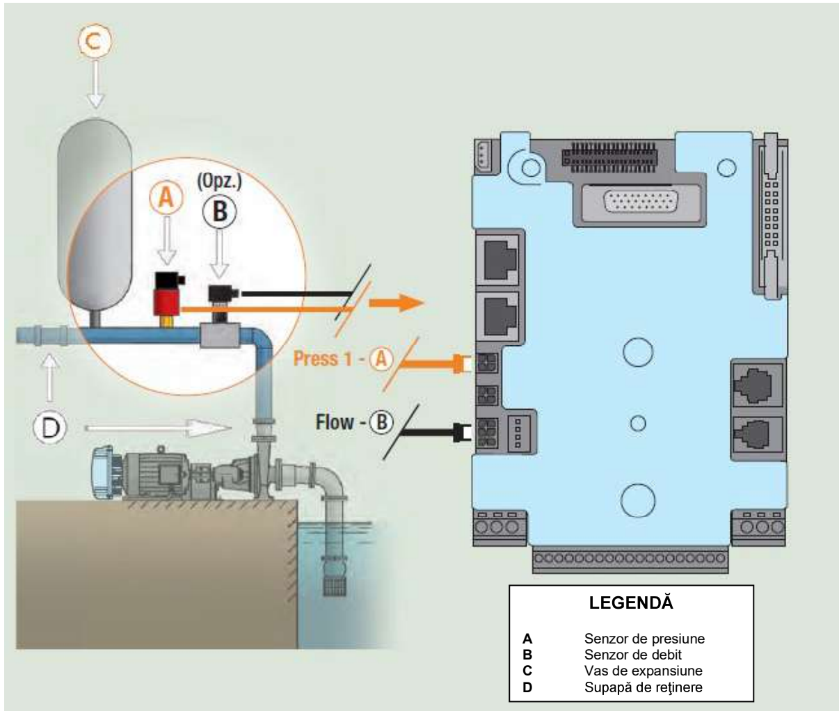
Figura 7: Instalația hidraulică
