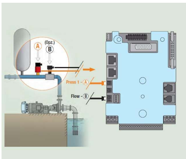
Figura 8: Conexiuni senzori
