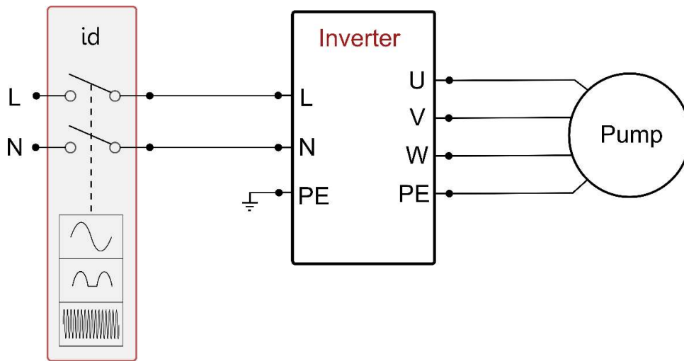
Figura 3a: Exemplu de instalare cu alimentare monofazică
