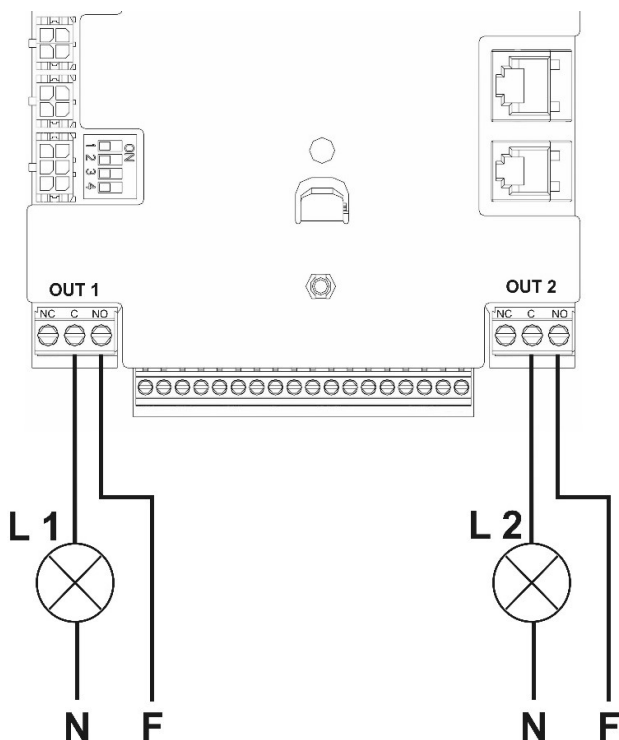
Figura 11: Exemplu de conectare a ieșirilor
