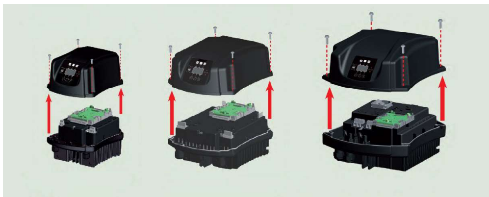
Figura 2: Demontarea capacului pentru accesul la conexiuni
