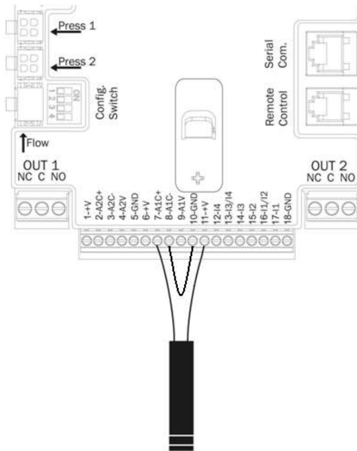
Figura 9: Conectarea senzorului de presiune 4 - 20 mA
