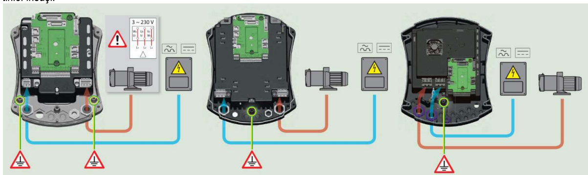
Figura 5: Conectări electrice
