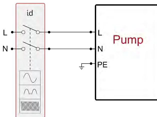
Kuva 11 esimerkki yksivaiheisesta asennuksesta
