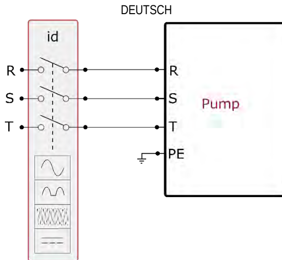
Abb. 2 Installationsbeispiel
