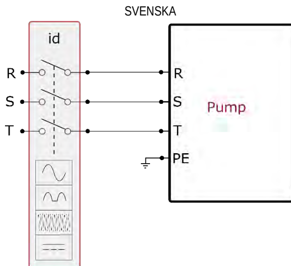
Fig. 12 Exempel på installation med trefasmatning
