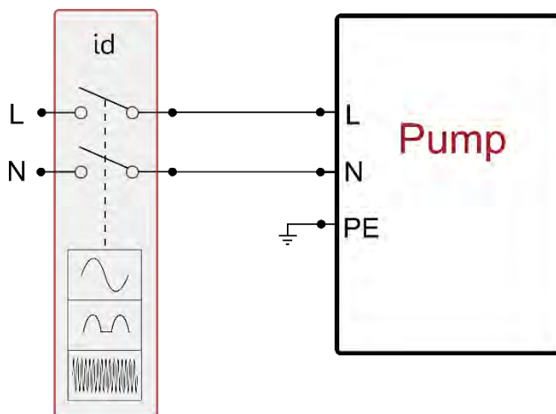
Фиг. 11 пример за инсталиране еднофазно
