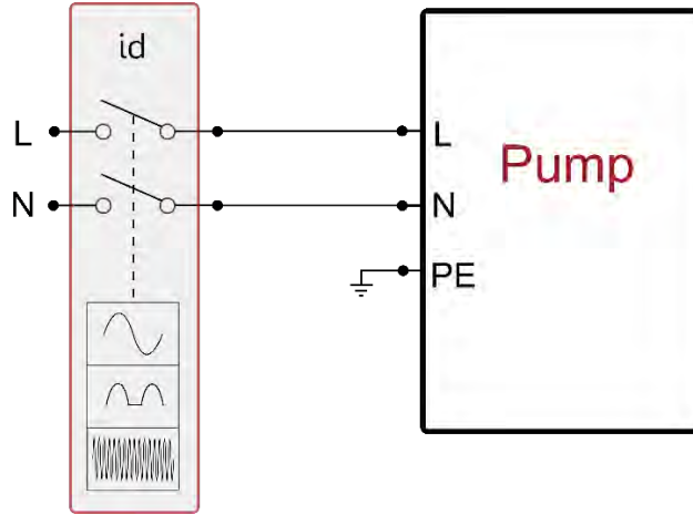
الشكل 11 مثال على التثبيت أحادي الطور
