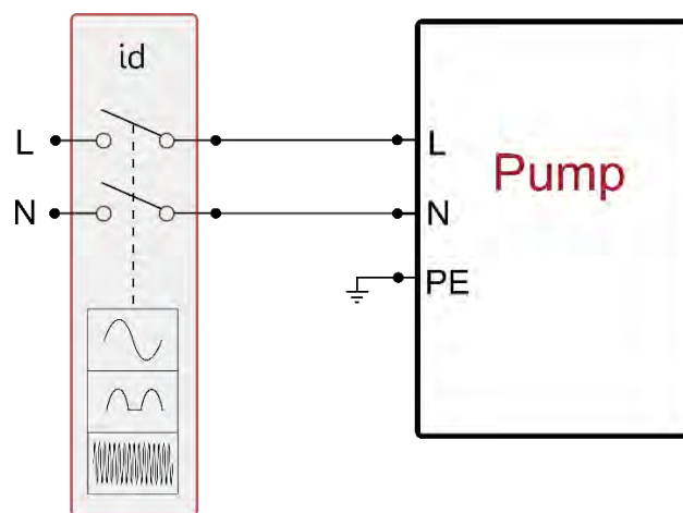
Afb 11 Installatievoorbeeld monofase
