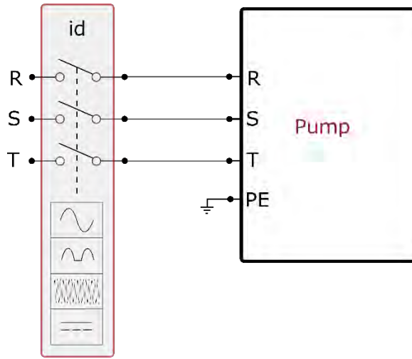
الشكل 12 مثال على التثبيت ثلاثي الطور
