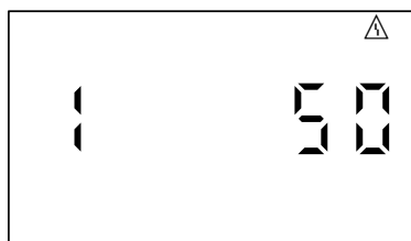
Fig. 42 Exemplu: Mesaj de avarie „50”
