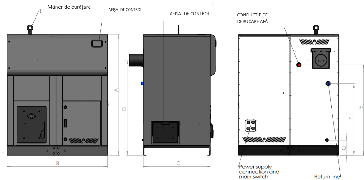
Figura 1. Cazan ECO MAX 35-100 (kW)
