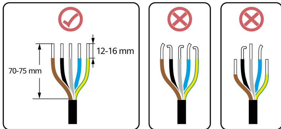
Figura 5-5 Cerințe de sertizare
