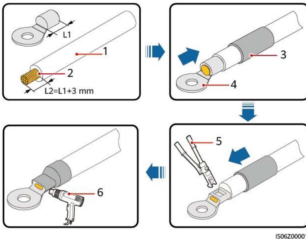
Figura 5-2 Sertizarea unei borne OT
