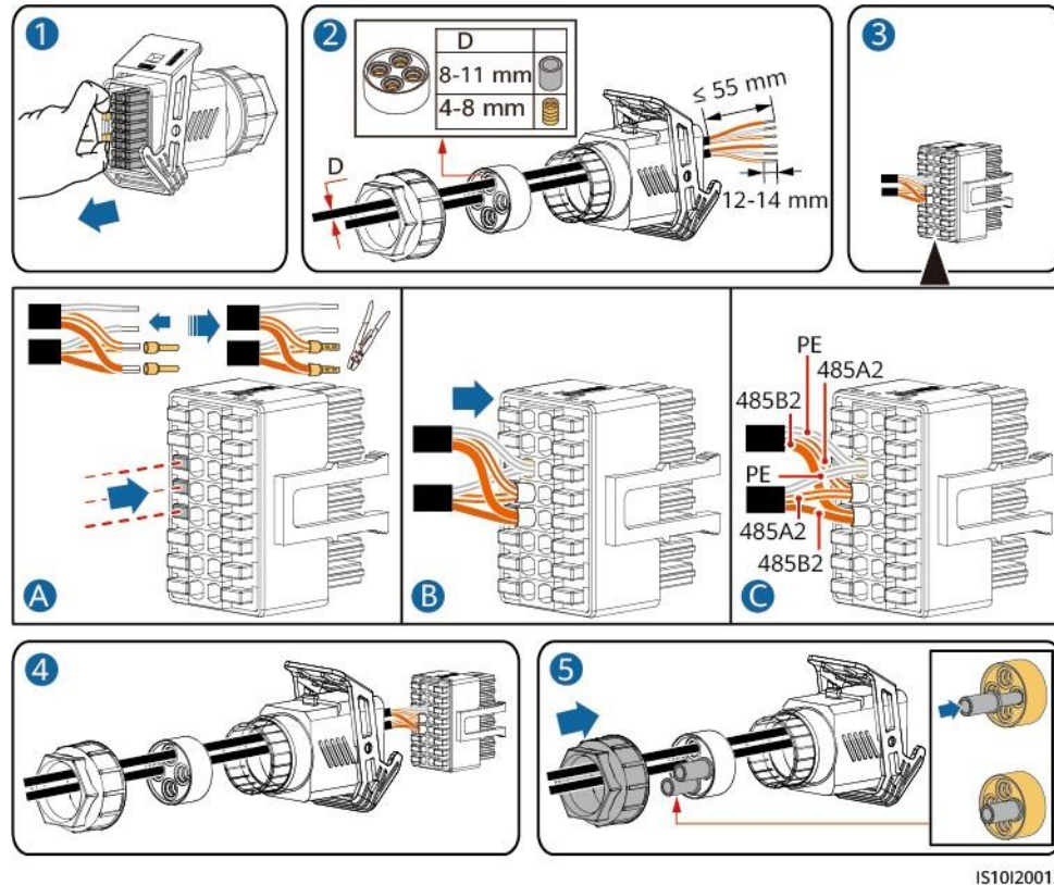
Figura 5-27 Instalarea cablului
