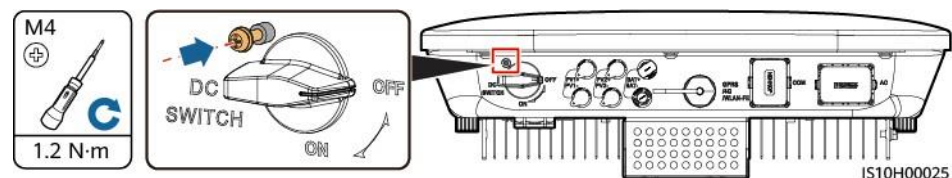
Figura 4-16 Instalarea unui șurub de blocare pentru întrerupătorul CC
