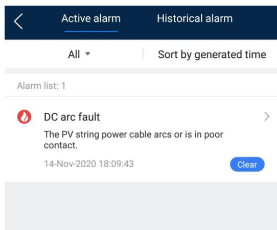
Figura 7-14 Managementul alarmelor
