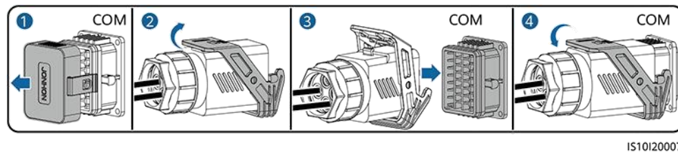
Figura 5-28 Fixarea conectorului cablului de semnal
