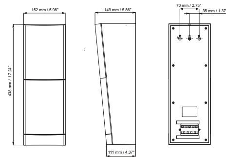
Fig. 4: Dimensions
